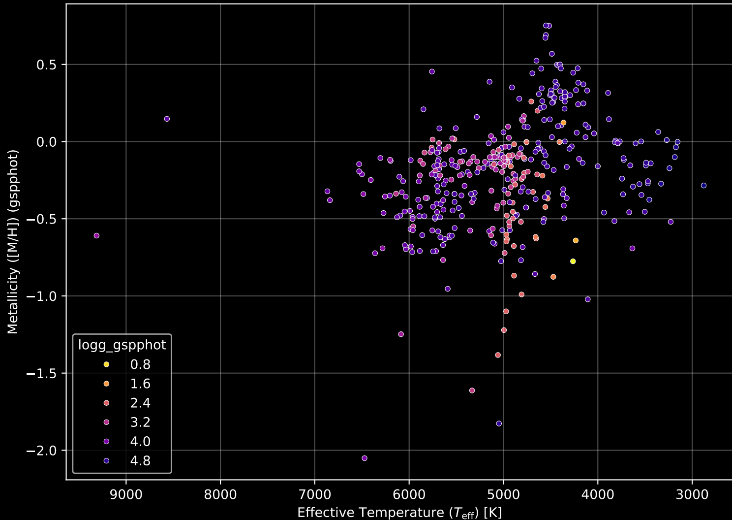
APOGEE DR17 Field: [000+60] Stellar Population Parameters (n= 392)
